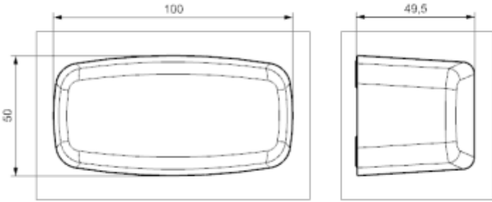
Şekil 1 : Radar Boyutları
